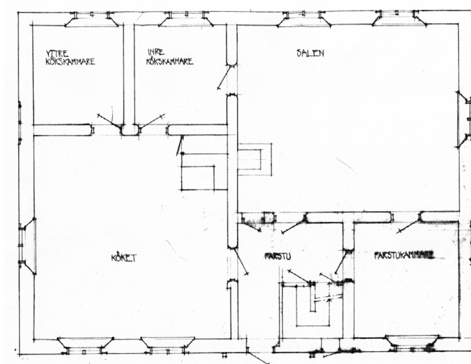
Planritning bottenvåningen (OBS, ritningen ej skalenlig)
